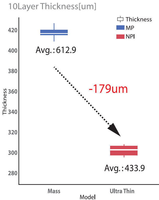
<10L THIN PCB_0.45T>
